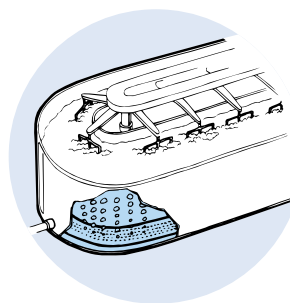
电镀液搅拌装置
