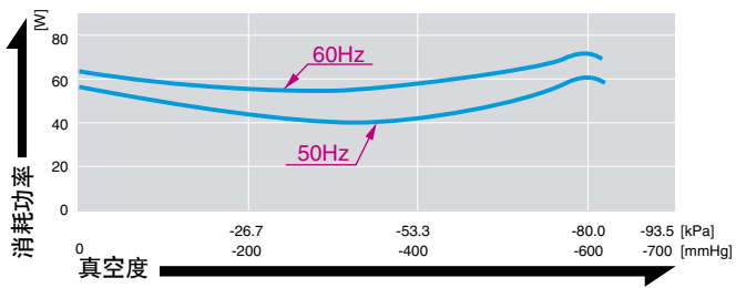
●消耗功率特性图
