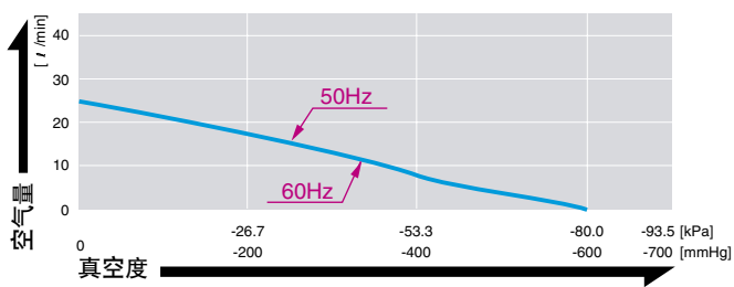
●空气量特性图
